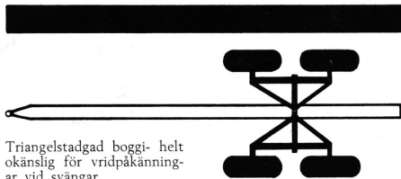
Bakbanke med boggi lätt flyttbar utefter distansstängan.
