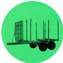
Rottne LP-boggi kan specialbyggas som griplastarvagn och utrustas med frontgrind och svansstyrning.
